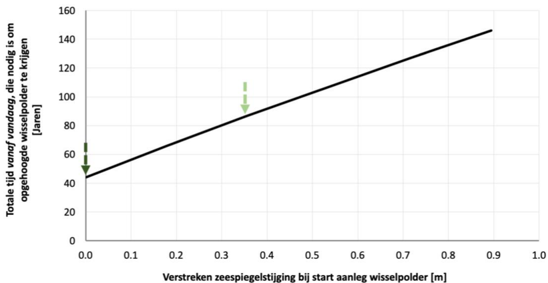
Figuur 3.7. Ontwikkeling van de bodemhoogte in de wisselpolder kost tijd. (A) wanneer direct wordt gestart dan kost het in een typische 30 – 50 jaar (in dit rekenvoorbeeld 44 jaar) om de gewenste hoogte te bereiken. Wordt de wisselpolder pas na 15 of 30 jaar geopend, dan heeft er meer relatieve zeespiegelstijging (incl. bodemdaling) plaatsgevonden waardoor het langer duurt om de gewenste bodemhoogte (target) te bereiken (respectievelijke 66 en 87 jaar). (B) Hoe langer zeespiegelstijging is voortgeschreden hoe langer er nodig is om de gewenste bodemhoogte te bereiken. De toename in benodigde extra tijd is 0,38 jaar per jaar uitstel wat overeenkomt met een extra 32 jaar tot target per 1 m relatieve zeespiegelstijging.
