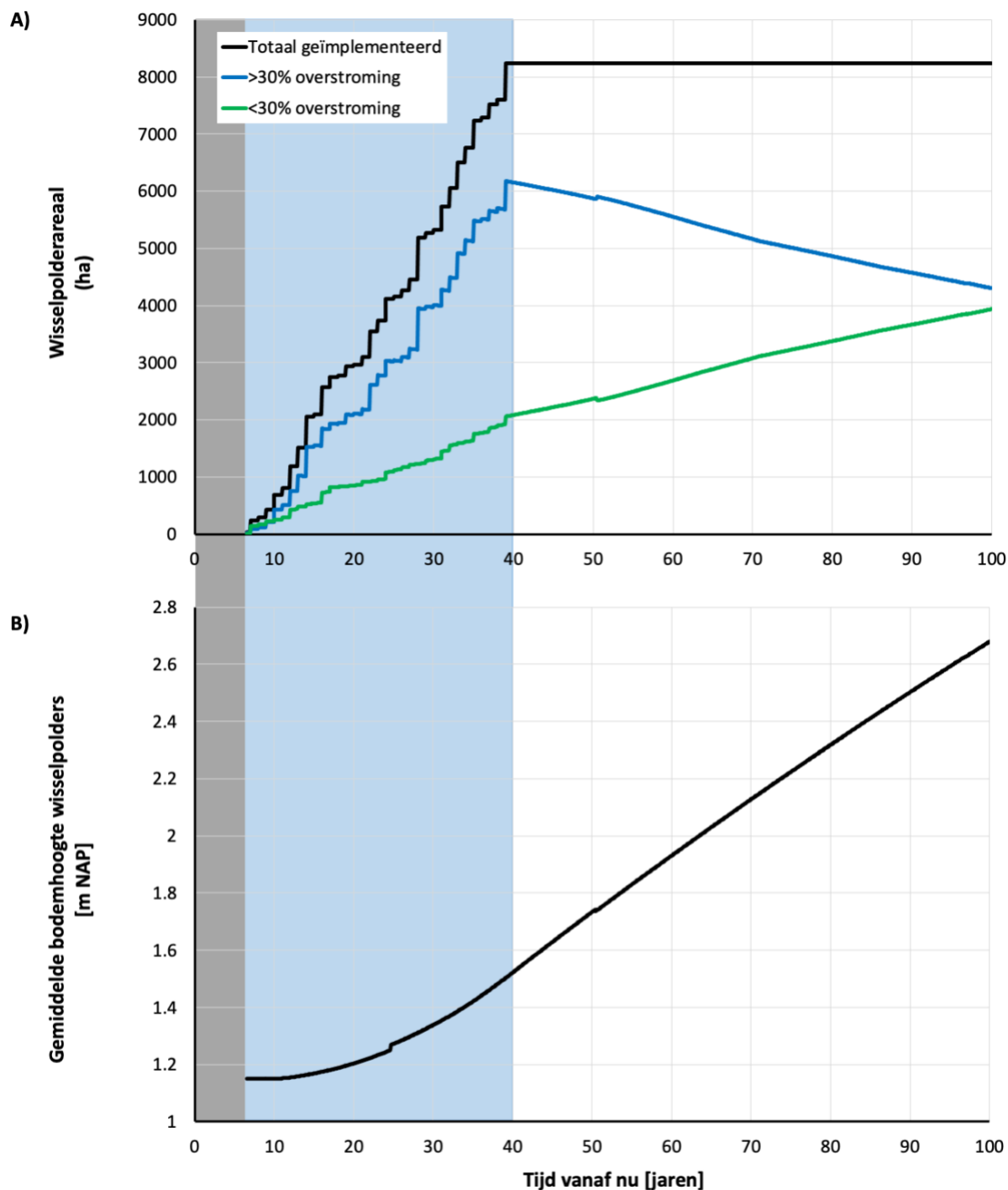
Figuur 3.6. Ontwikkeling van het areaal (A) en bodemhoogte (B) over de tijd voor de polders in het potentiële dubbele dijken met wisselpolders langs de Westerschelde. Ontwikkelingen bij een verwachte zeespiegelstijging van 1 m in 2100. Dubbele dijken worden over een periode van 40 jaar geïmplementeerd (blauwe zone) met een voorbereiding van 5 jaar (grijze zone)
